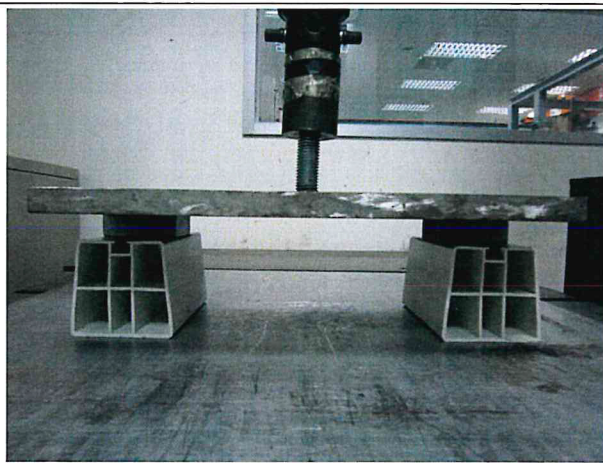
照片 B：測試架設
