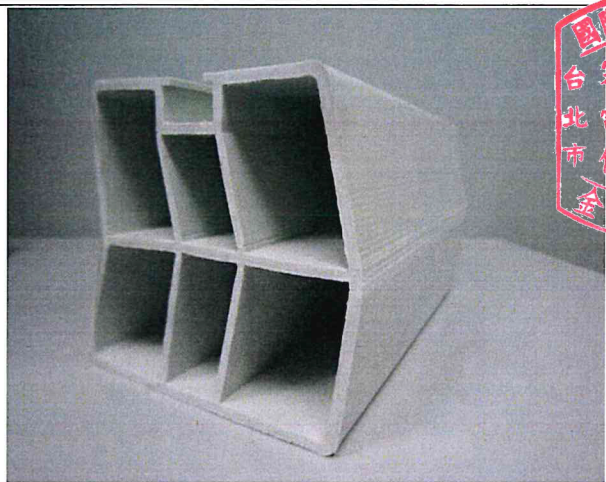
照片 C：測試後樣品外觀
